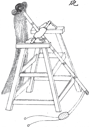
图五 北宋《武经总要》描绘的单梢砲
